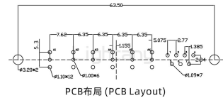
PCB布局 (PCB Layout)
