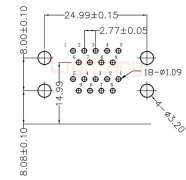
PCB布局 (PCB Layout)
