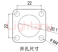
开孔尺寸
